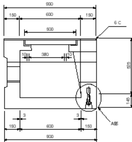
中央断面図
