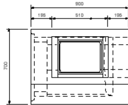
中央断面図
